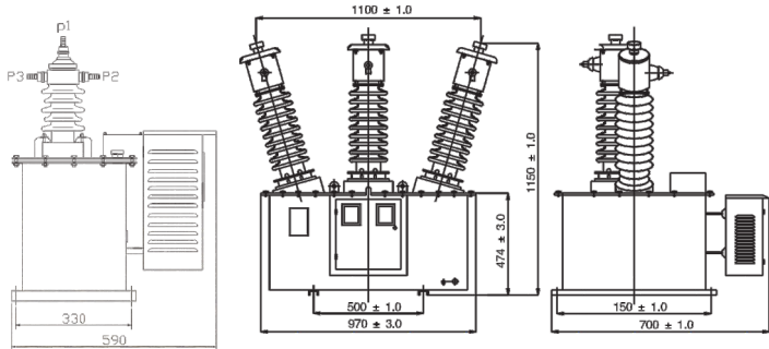
JLS4-35
