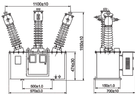
JLS-35
