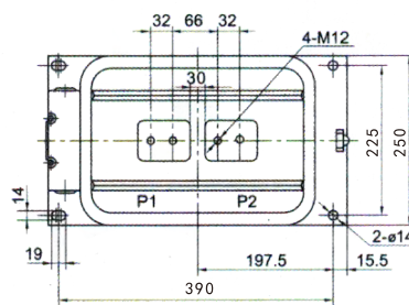
20-1250A K 向 Direction K
