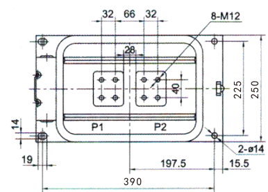
1500-2500A K 向 Direction K
