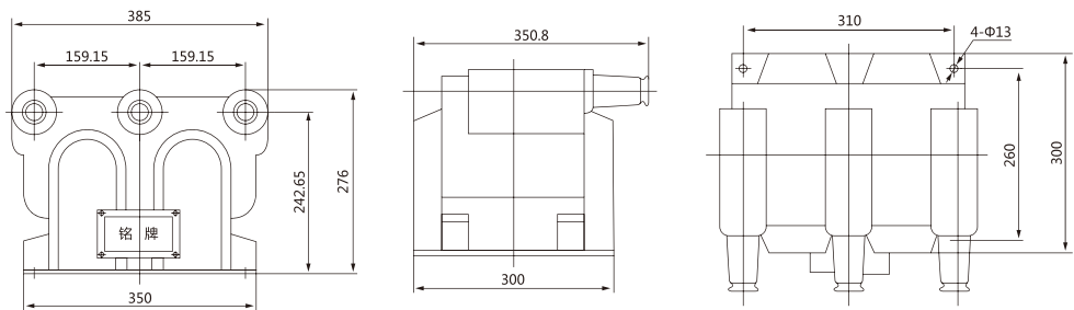
JSZV12-10R
