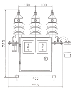
JLS4-10
