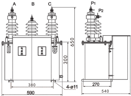
JLS-6、10
