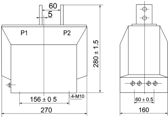
LZZBJ9-10
