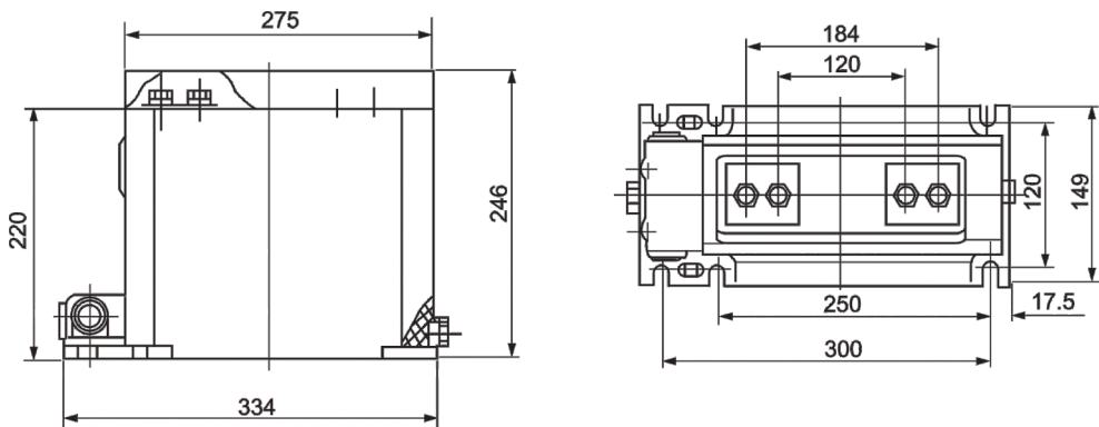
LZZBJ9-12(AS12/150b2S)
